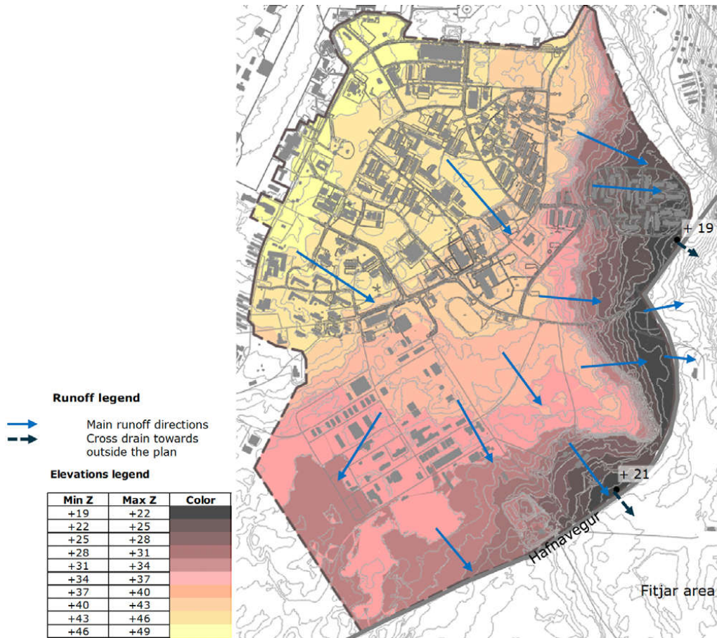
Mynd 2.2. Landhæð og meginrennislíleiðir ofanvatns. Kort úr skýrslu COWI um blágrænar ofanvatnslausnir á Ásbrú.
